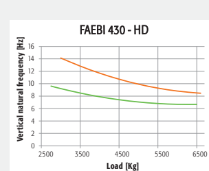
FAEBI® 430-HD
